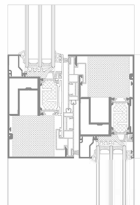
przekrój przez połączenie skrzydła-skrzydło (UG 820 + UG 830)
