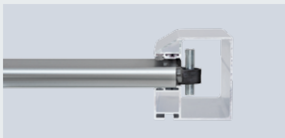
Brama rolowana DD profil Decotherm S ze stalowymi hakami przeciwwiatrowymi (w bramach o szerokości lub wysokości powyżej 5000 mm lub opcjonalnie przy wyższych wymaganiach dotyczących odporności na obciążenie wiatrem)
